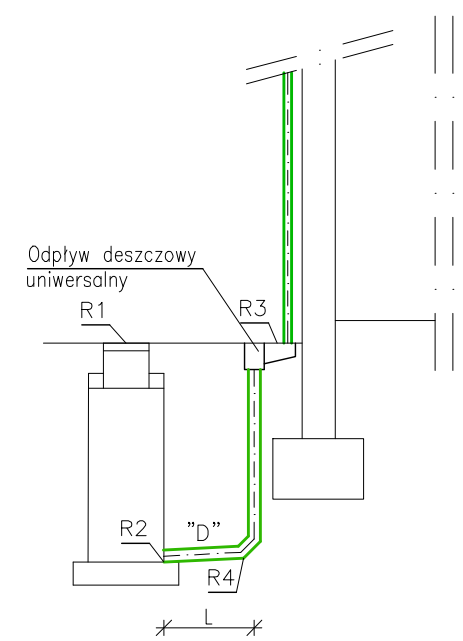
Szczegół przykanalika do rury spustowej
